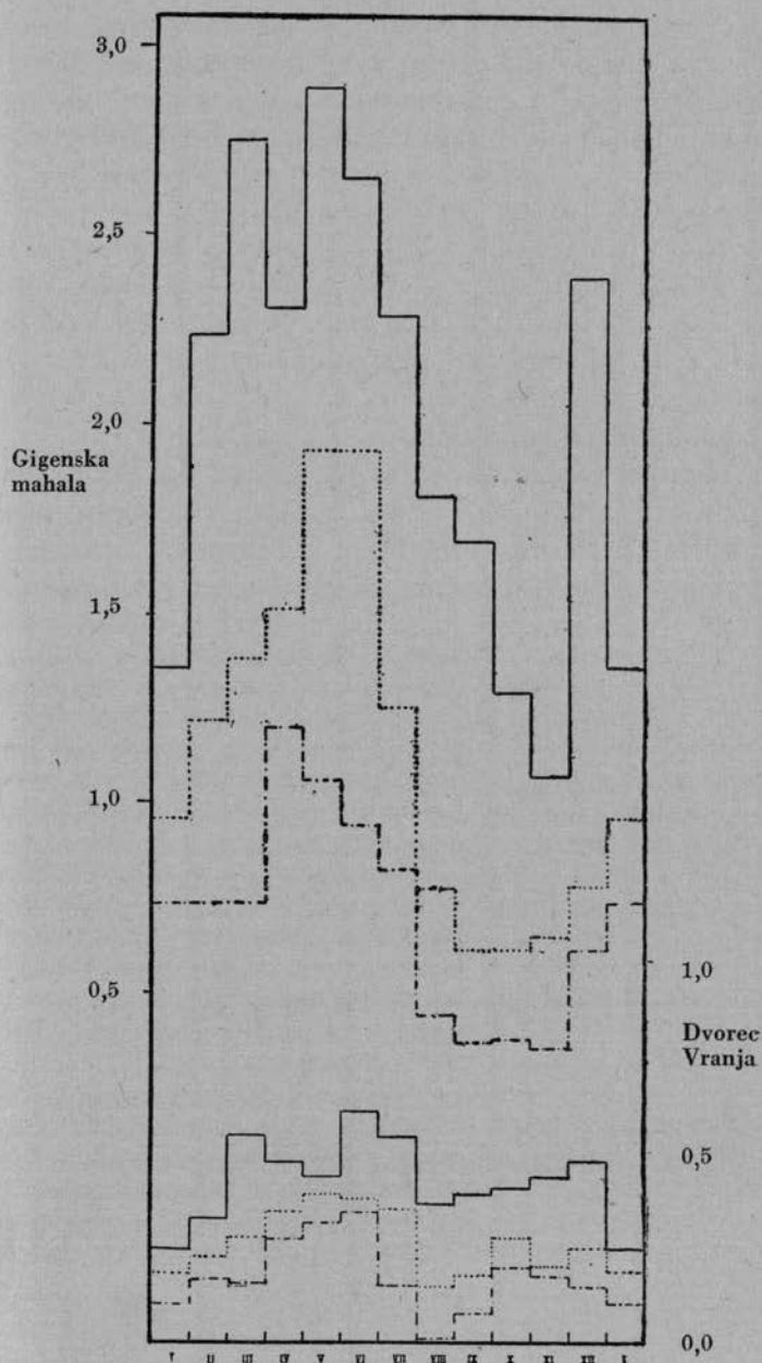
DIAGR. XVII. — Oscillazioni medie di livello dell'Iskär a Dvorec Vranja (a destra) ed a Gigenška mahala (a sinistra).
