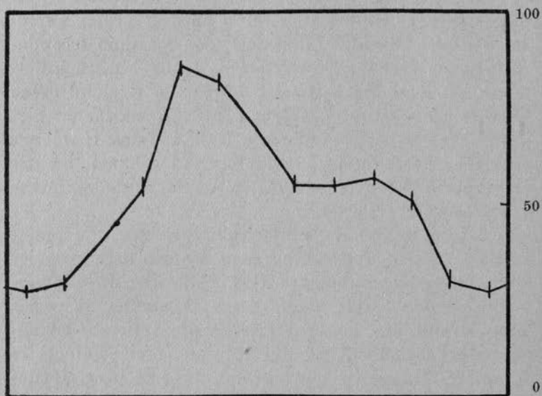
DIAGR. VII. — Andamento mensile medio delle precipitazioni a Sofia.
