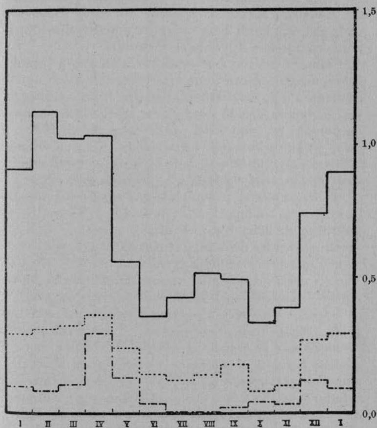
DIAGR. XXVIII. — Oscillazioni medie di livello del Tundža a Šablii.
