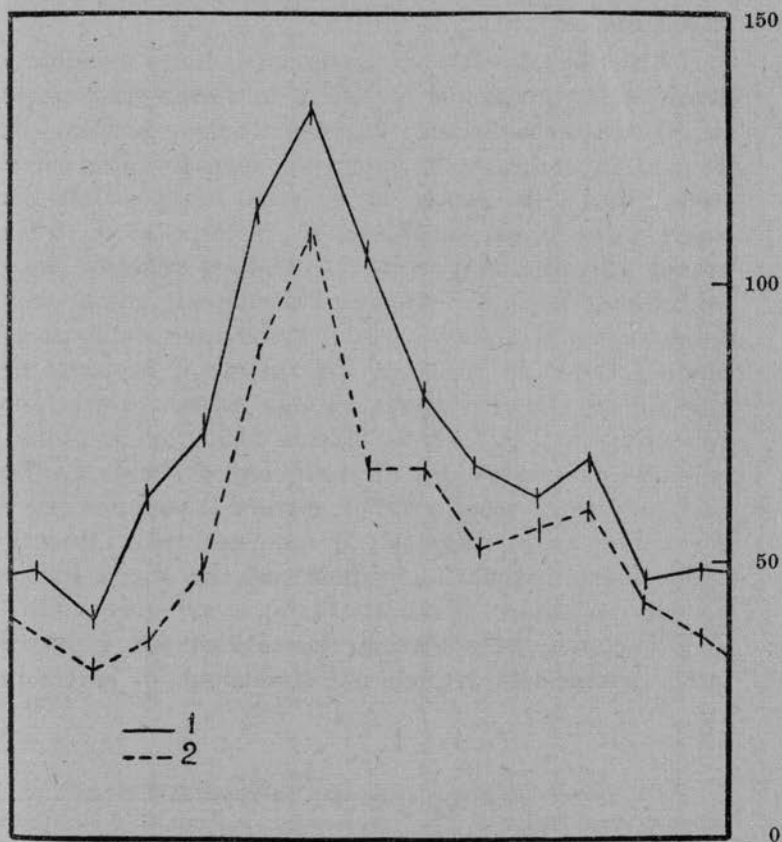
DIAGR. II. — Andamento mensile medio delle precipitazioni a 1. Gabrovo; 2. Kazanlak.
