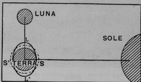
Formazione delle maree.
