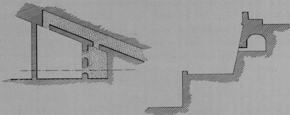
FIG. 325 — SCHIZZO DI PIANTA E SPACCATO DEL FIANCO DEL BALUARDO MARTINENGO.
