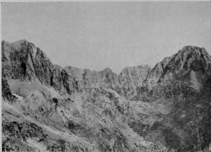
Vista dalla Jesera verso i monti Papluk.
