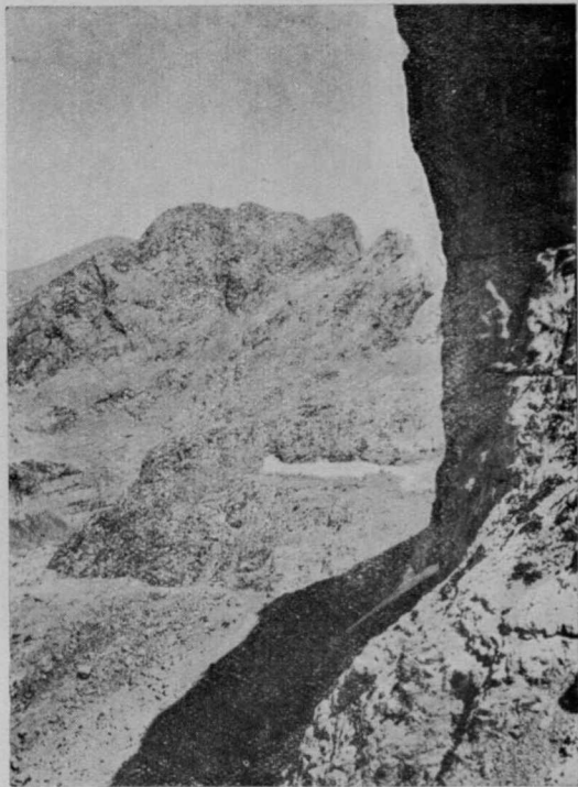
Terrazze e gole di lisciamiento in una valle sorgente della Jesera.
