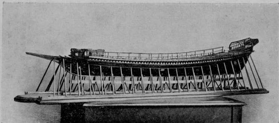
N° 900. — Galère ordinaire sur son chantier.
