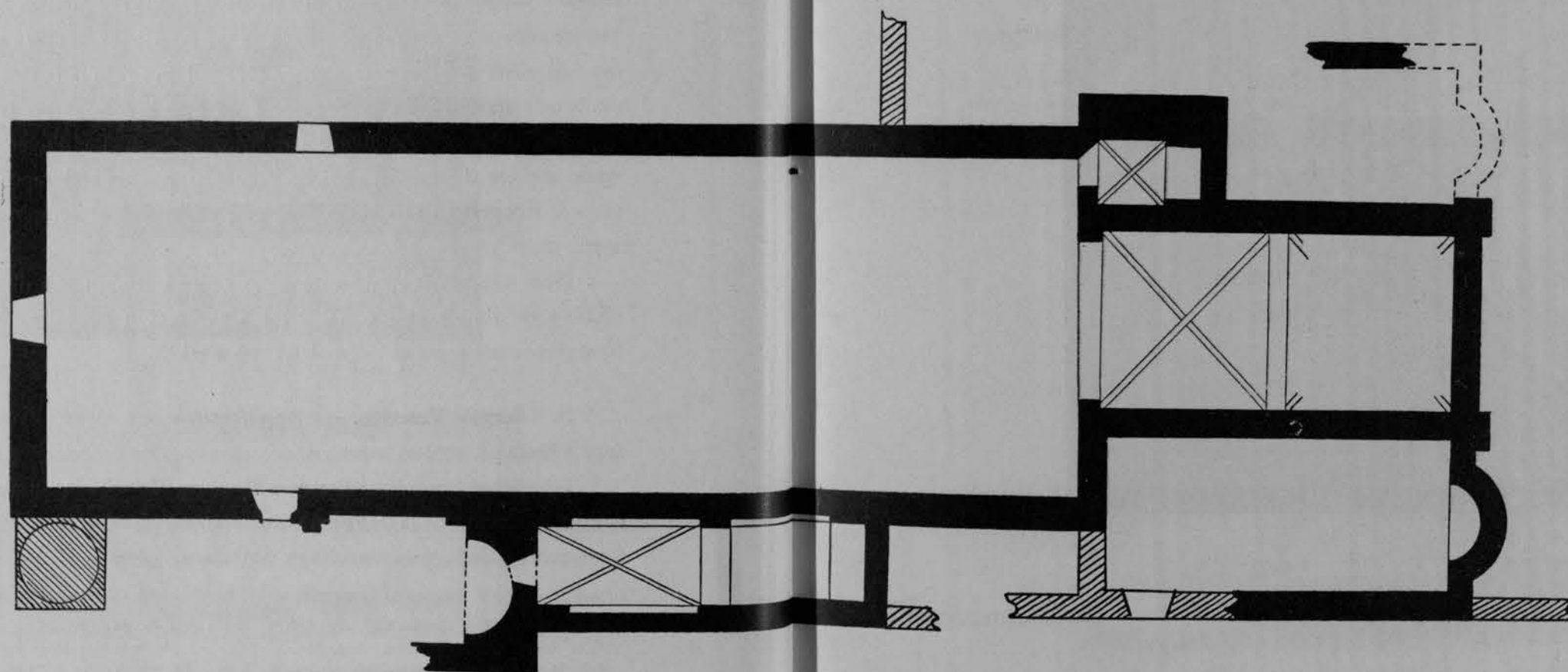
FIG. 74 — PIANTE DELLA CHIESA DI S. SALVATORE A CANDIA.
