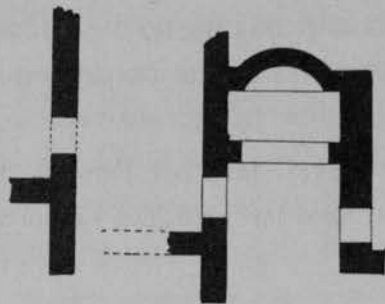
FIG. 18 — PIANTE DELLA CHIESA DI SANTA DOMENICA PRESSO *ARGHJIRÚPOLIS.
