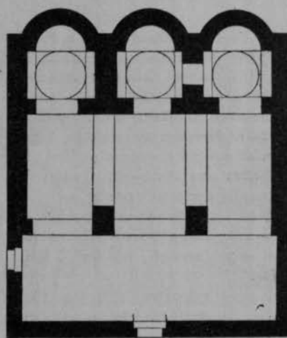
FIG. 279 — Pianta della Chiesa di S. Maria a *Kji-tharidha (Malvesin).
