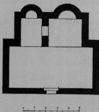
FIG. 274 — Pianta della Chiesa di S. Maria al Convento di Gerusalemme (Malvesin).
