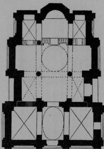
FIG. 273 — Pianta della Chiesa di San Chirgiani presso *Alíkjanù (Canea).
