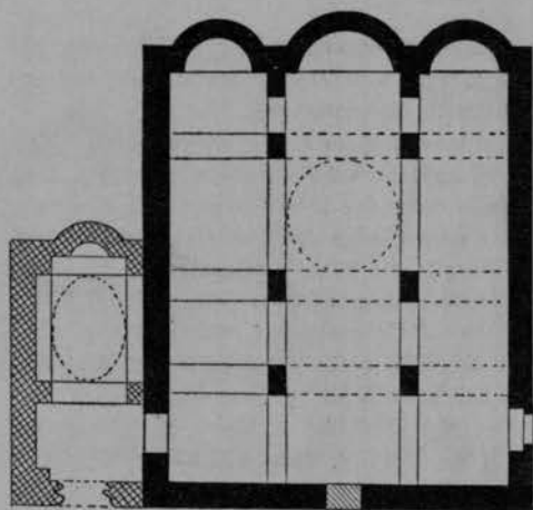
FIG. 277 — Pianta della Chiesa della *Kjerà presso *Asòmato (Amari).
