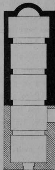
FIG. 22 — PIANTA DELLA CHIESA DI S. SALVATORE A * ŽEVREMJANÀ.
