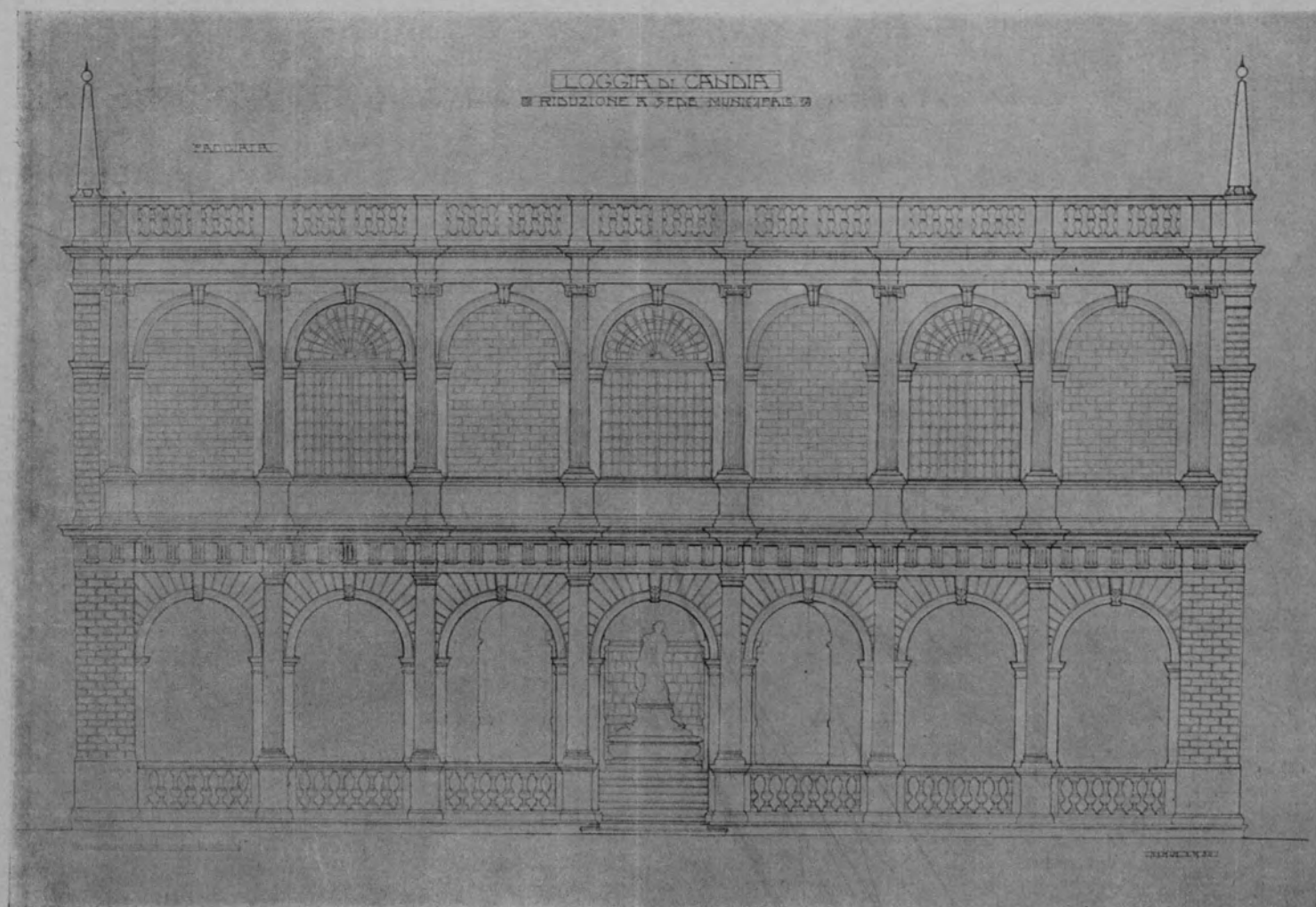
FIG. 10 — PROGETTO ONGARO DI RICOSTRUZIONE DELLA LOGGIA DI CANDIA.
