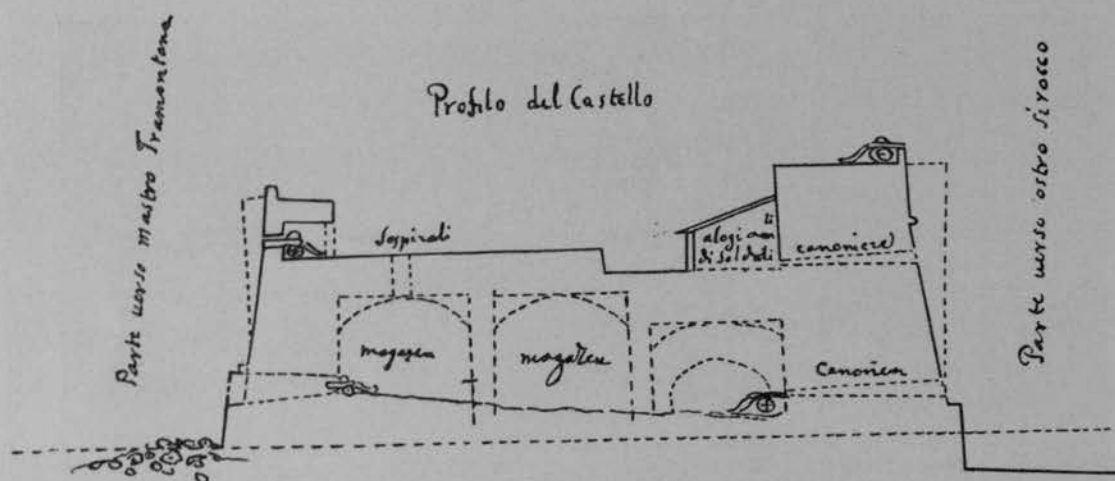
FIG. 70 — SPACCATO DELLA ROCCA A MARE DI CANDIA — SECOLO XVII — (LIV. a.).
