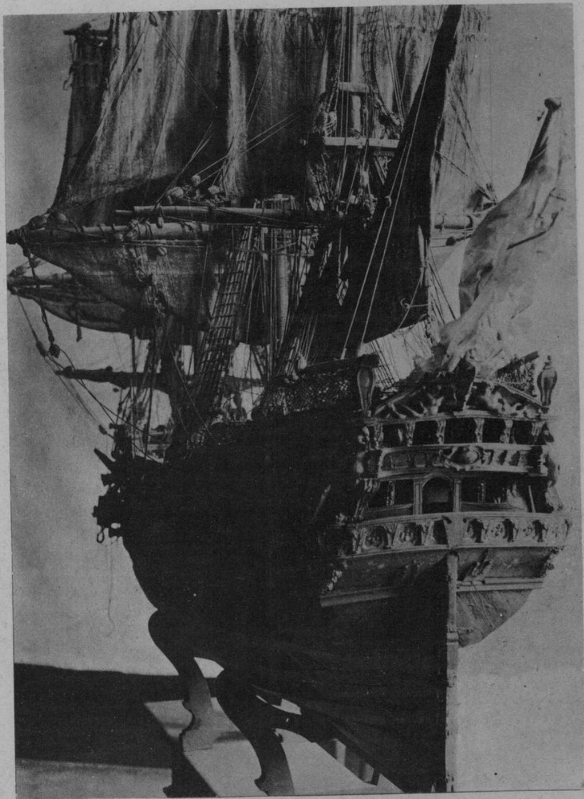
Fig. 202 - Il modello del vascello S. Antonio visto da poppavia. (vedi figure n. 201 e 208)
