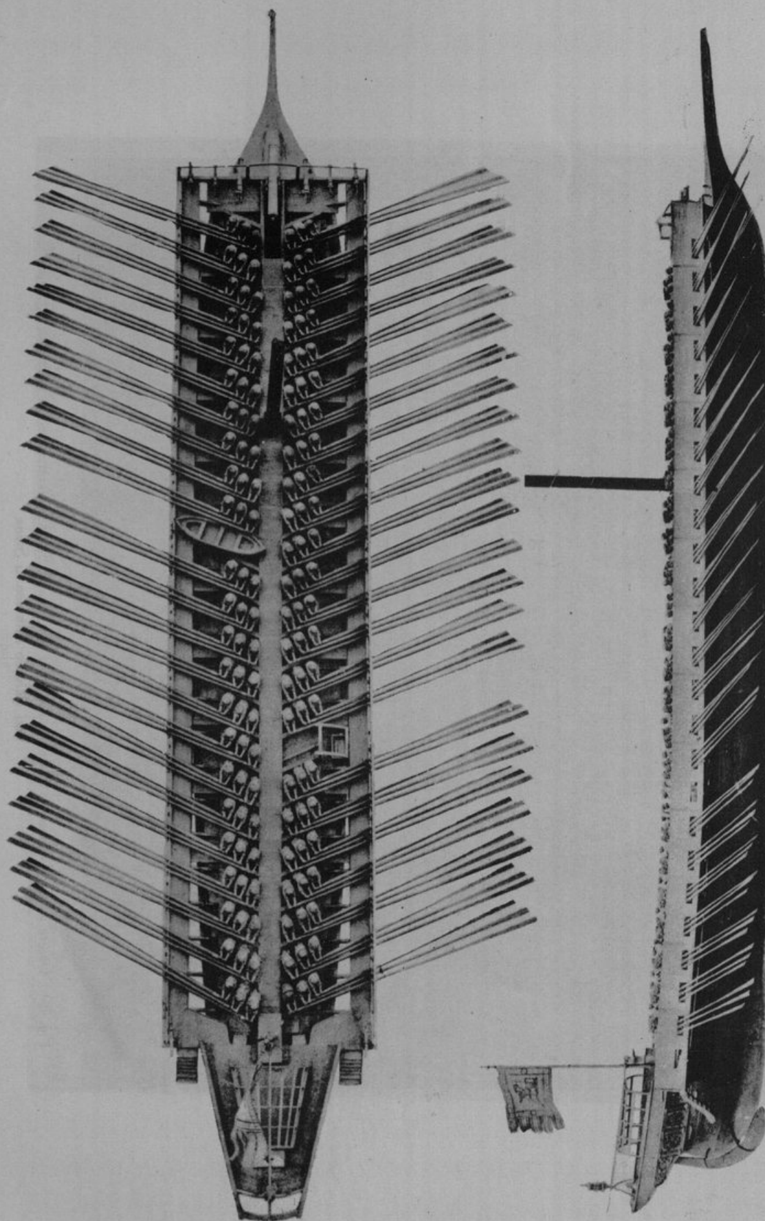
Fig. 29 - Galera veneta "alla sensile" vista dall'alto e di profilo, colla disposizione dei banchi di vogha, dell'apposticcio, della rembata e delle altre parti. Dal modello della trirème del 1539 dell'Ammiraglio Fincati al Museo Navale di Venezia.
