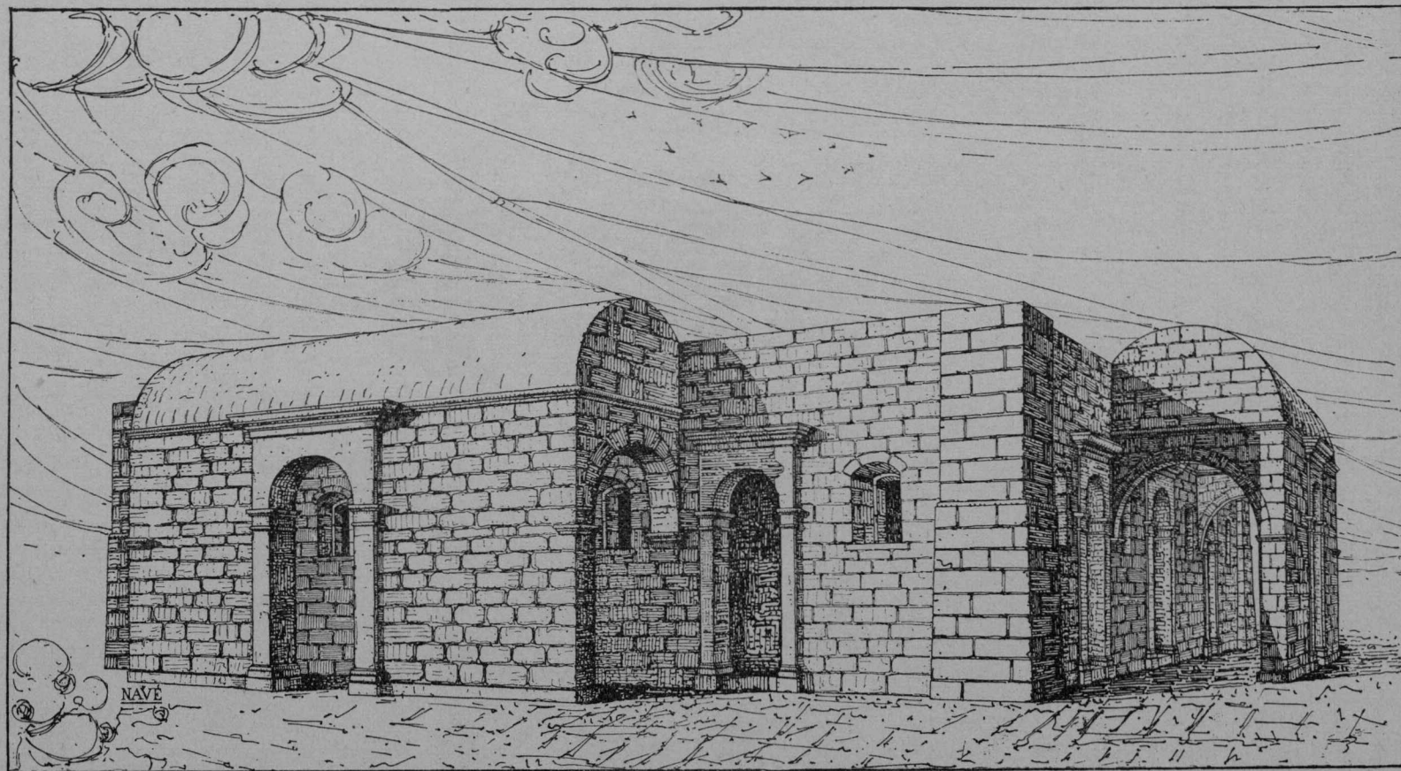
FIG. 155 — RICOSTRUZIONE GRAFICA DELLA *RETÓNDA DI *KALÁTHENES.
