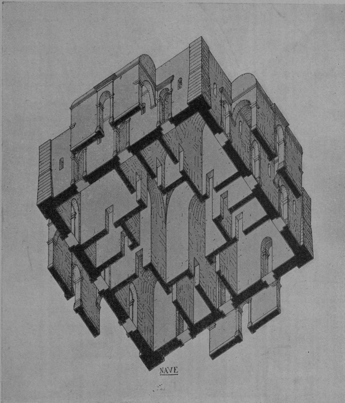
FIG. 154 — PIANTE E RICOSTRUZIONE GRAFICA DELLA * RETÓNDA DI * KALÁTHENES.
