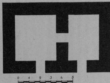
FIG. 59 — PIANTA DELL'ALTRA POLVERIERA DI RETIMO.
