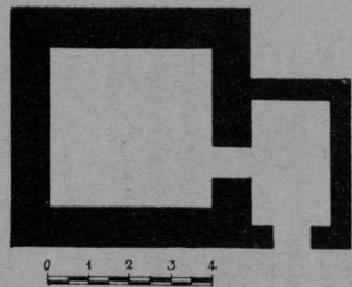
FIG. 57 — PIANTA DI UNA POLVERIERA DI RETIMO.
