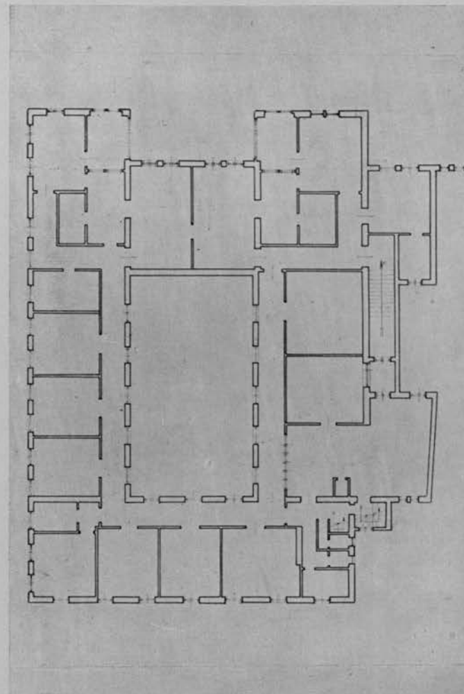
183 - Pianta del secondo piano del palazzo di Venezia (stato attuale).
