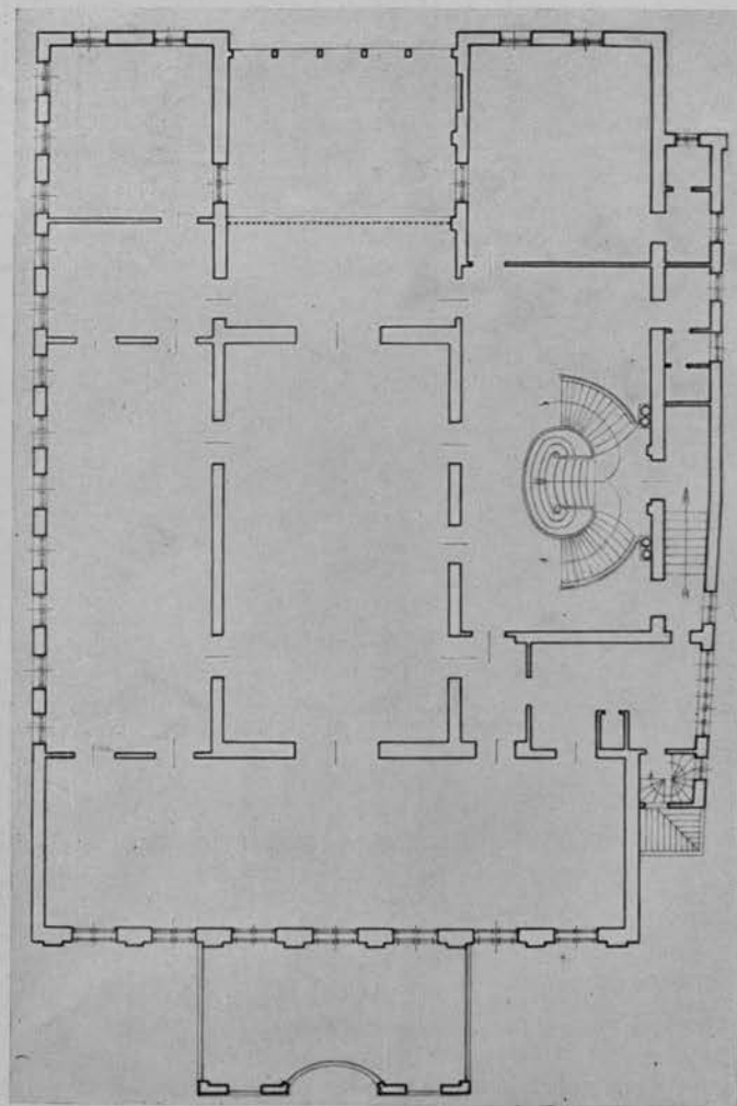
182 - Pianta del primo piano del palazzo di Venezia (stato attuale).
