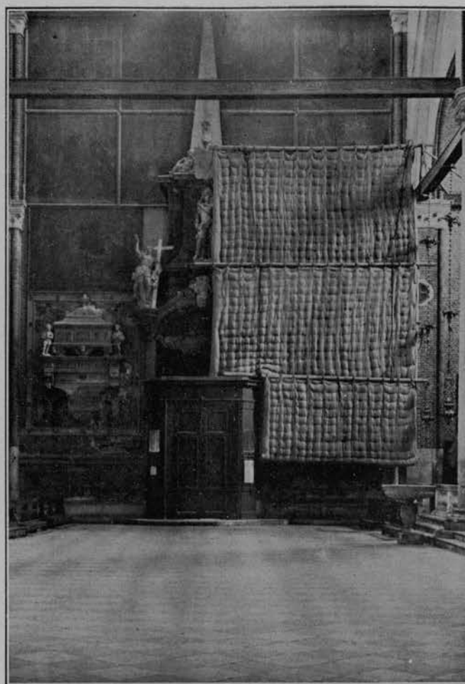
CHIESA DEI FRARI PROTEZIONE CON MATERASSI PARA-SCHEGGE
