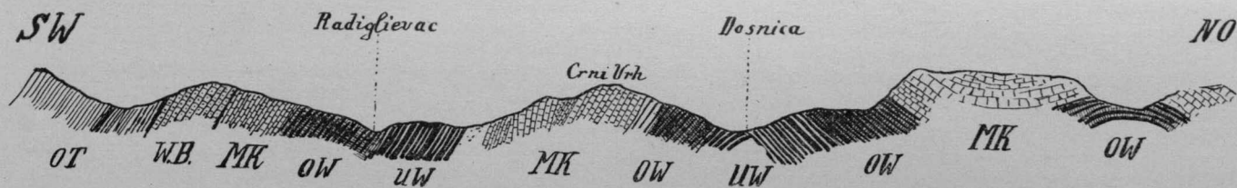
Sl. 108. Prosjek kroz Crni vrh od sjeveroistoka prema jugozapadu. U W = donje verfenske naslage, O W = gornje verfenske naslage, MK = ljuštuno vapno, B W = buhensteinske i vengenske naslage, O T = gornji trias.
